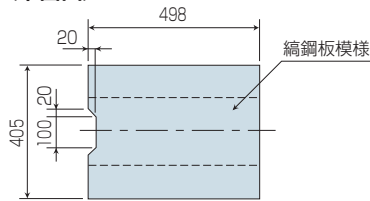
〔側面図〕
