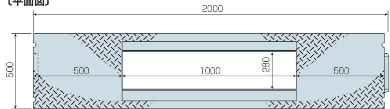
〔平面図〕
