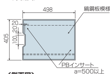
〔側面図〕
