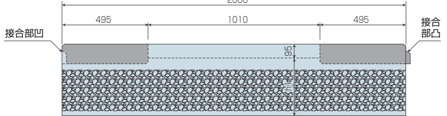
〔側面図〕
