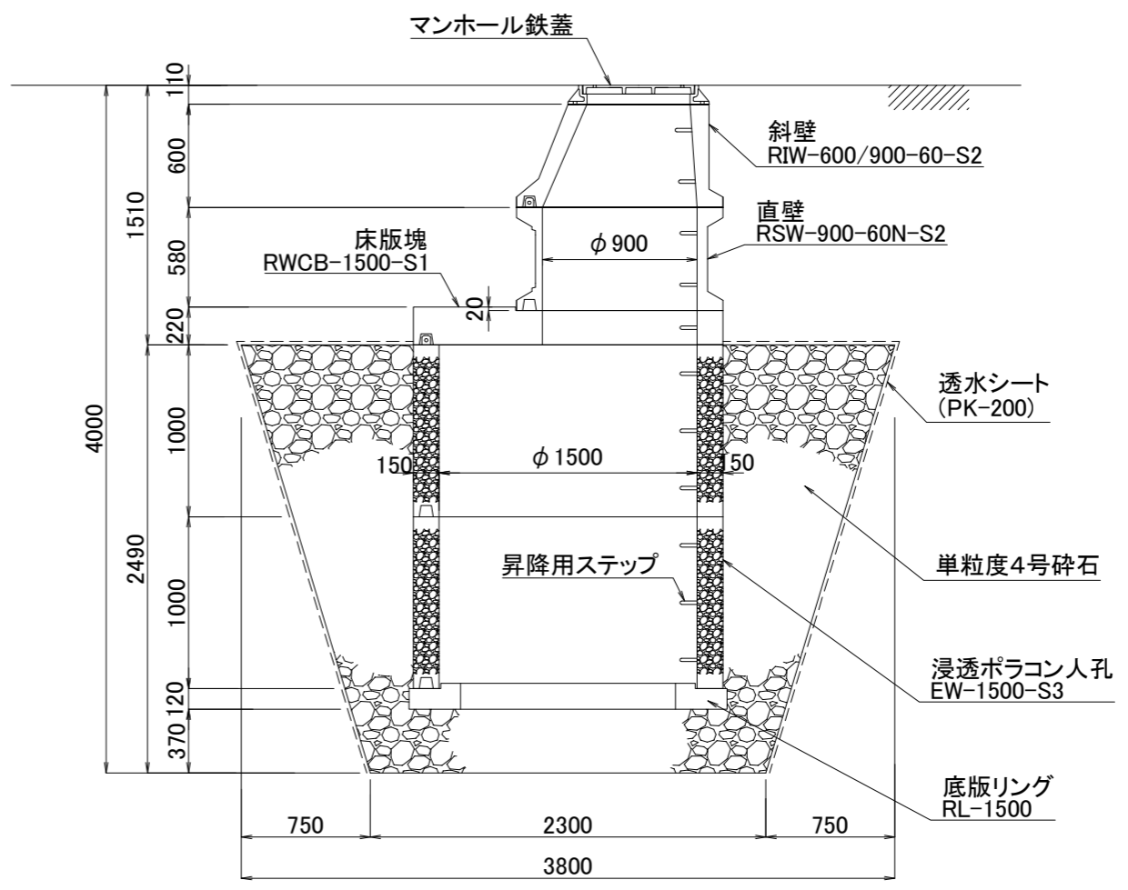
断面図
