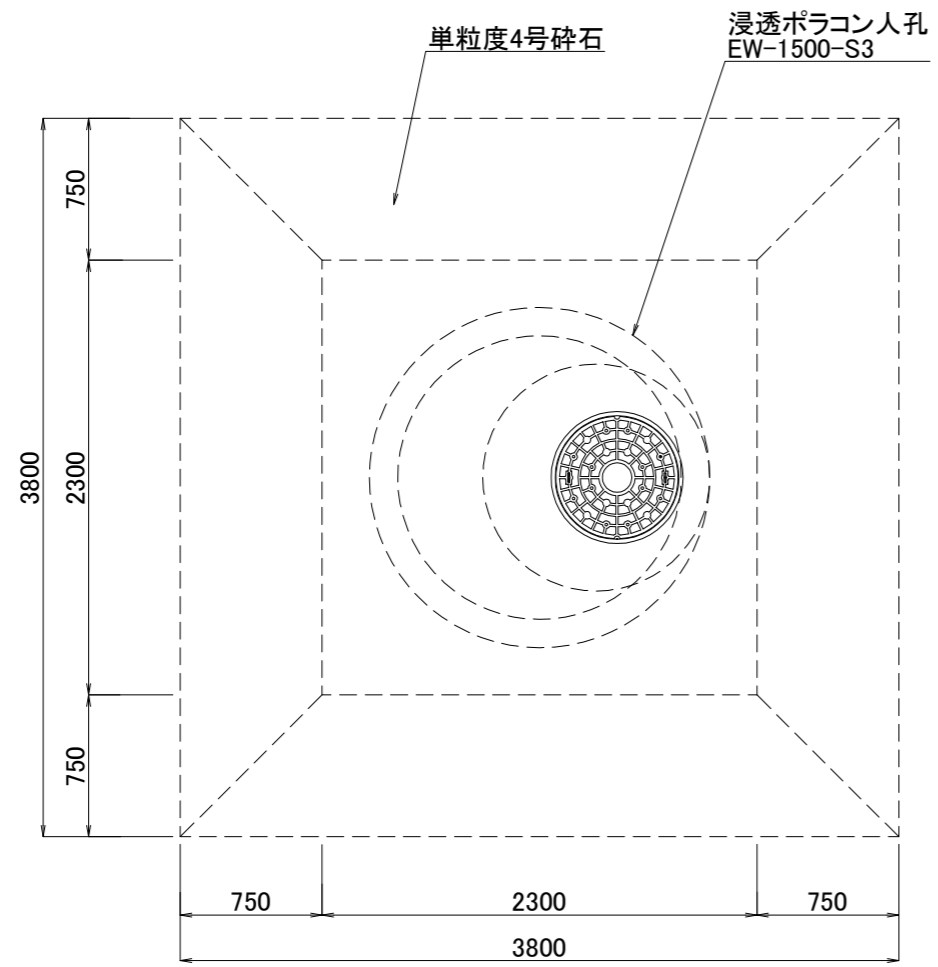
平面図
