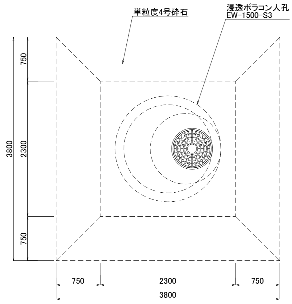
平面図
