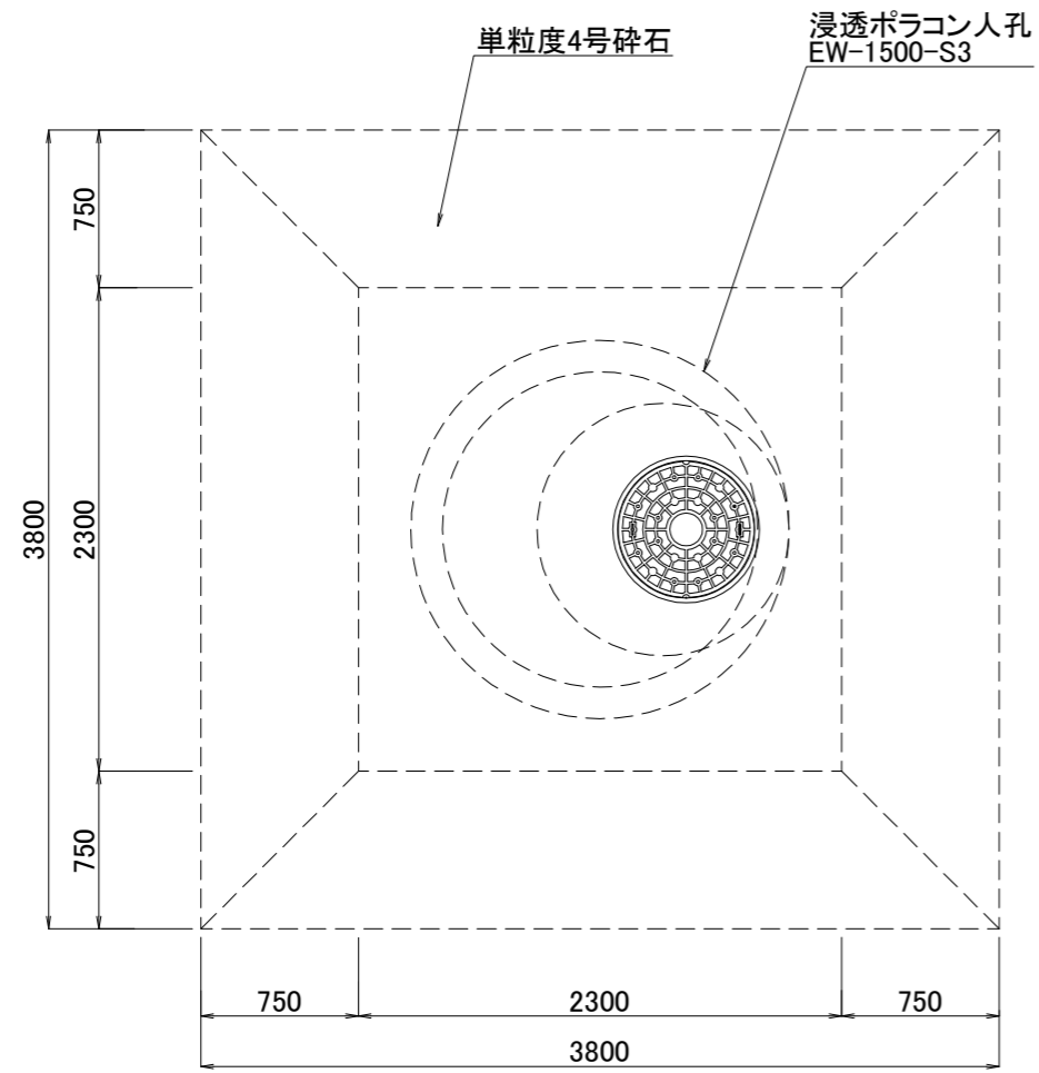
平面図
