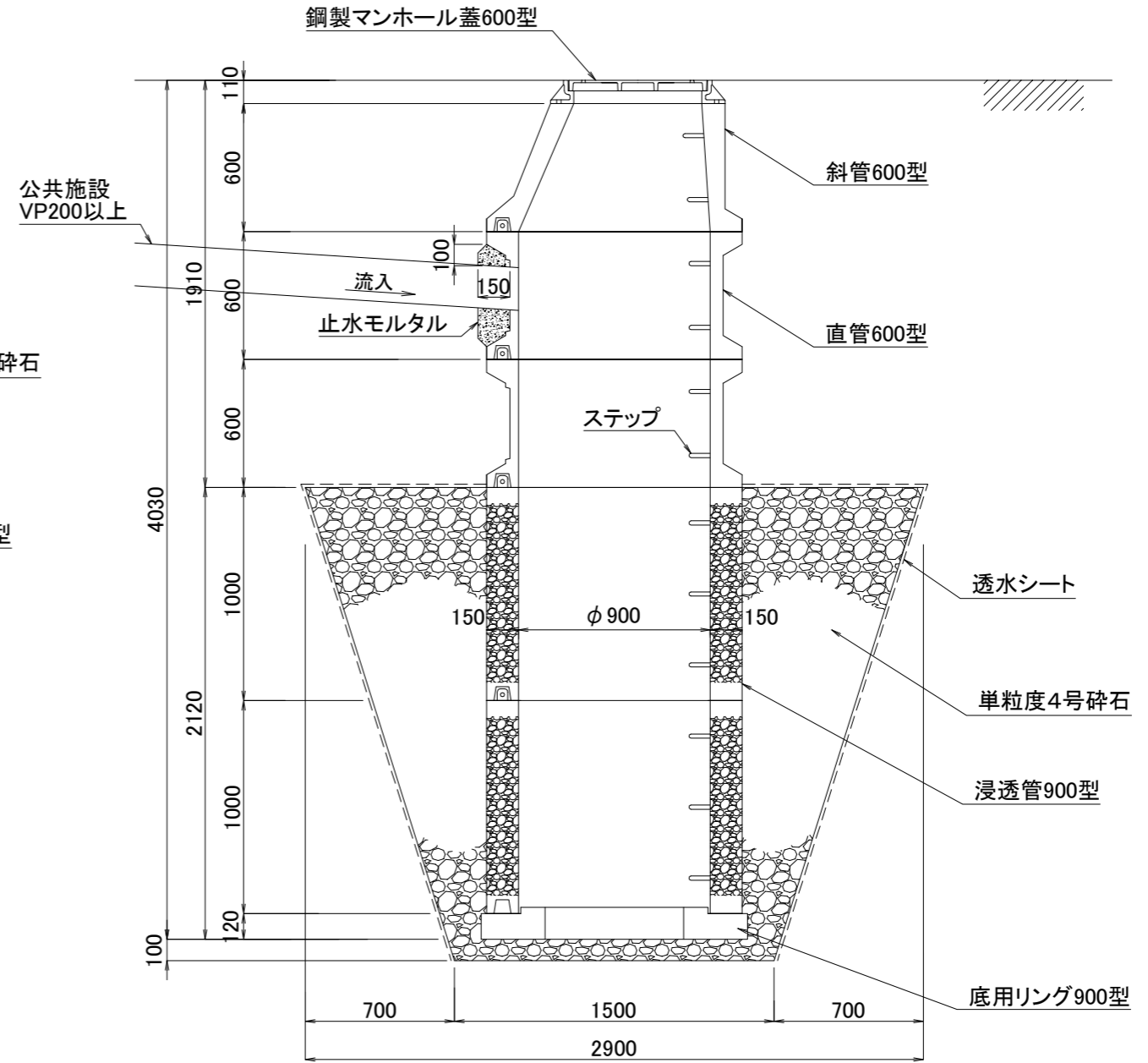
断面図
