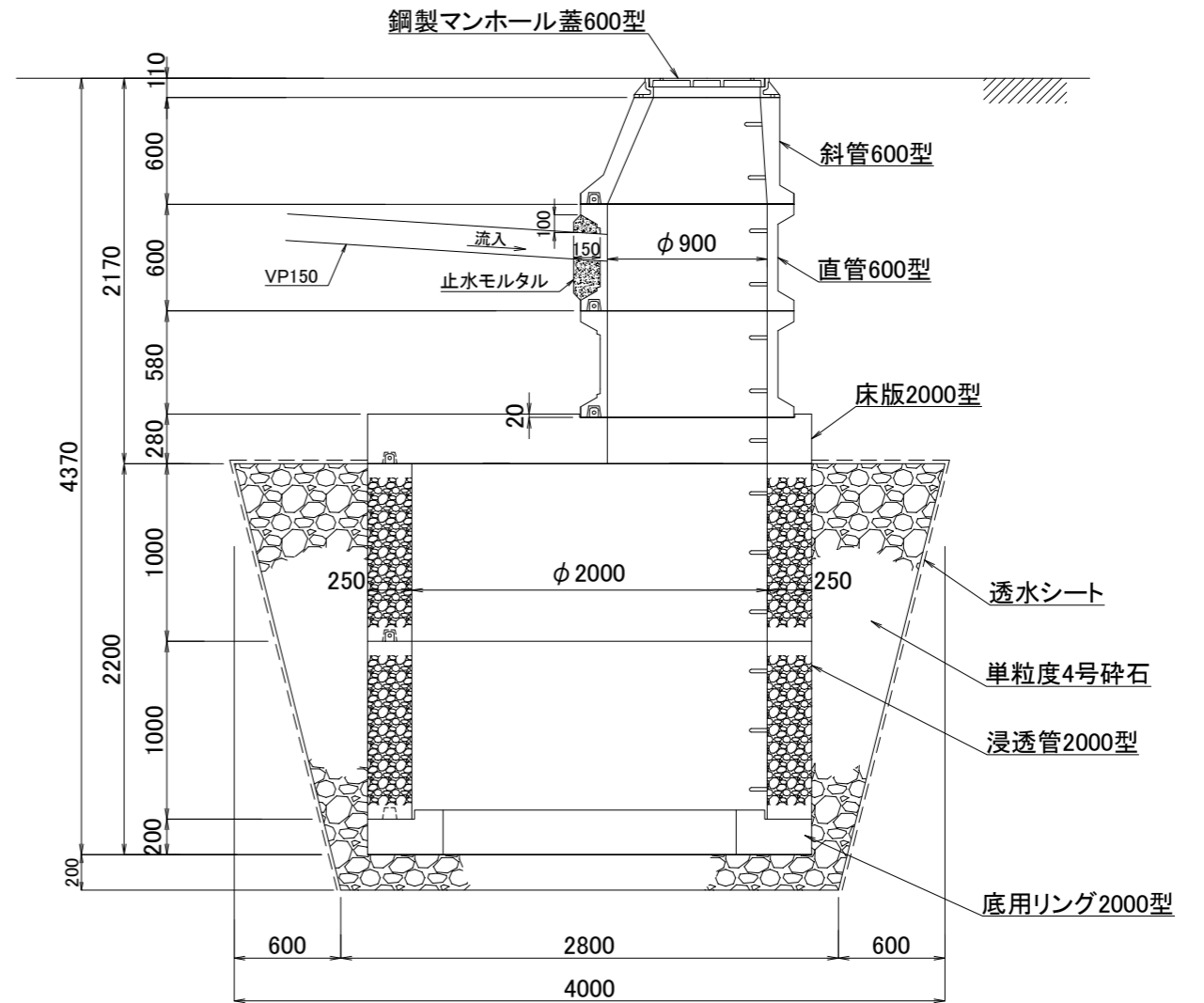
断面図
