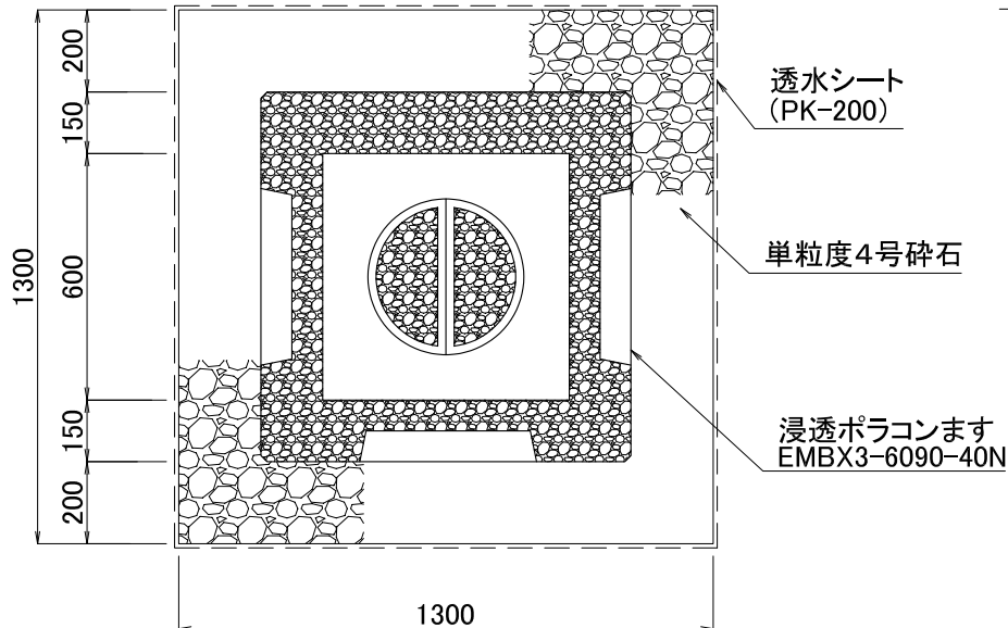
柵底部
