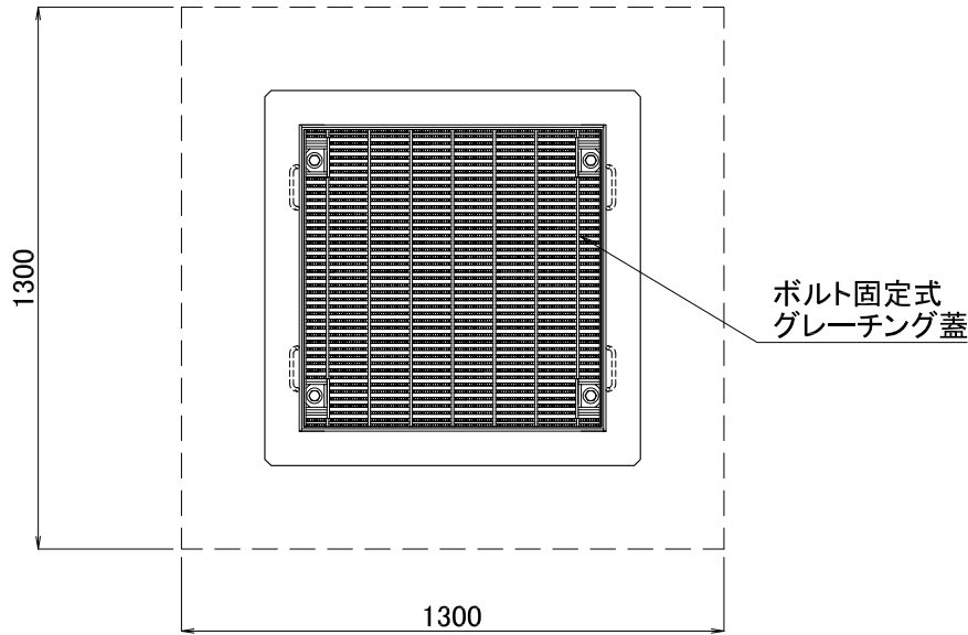
柵底部
