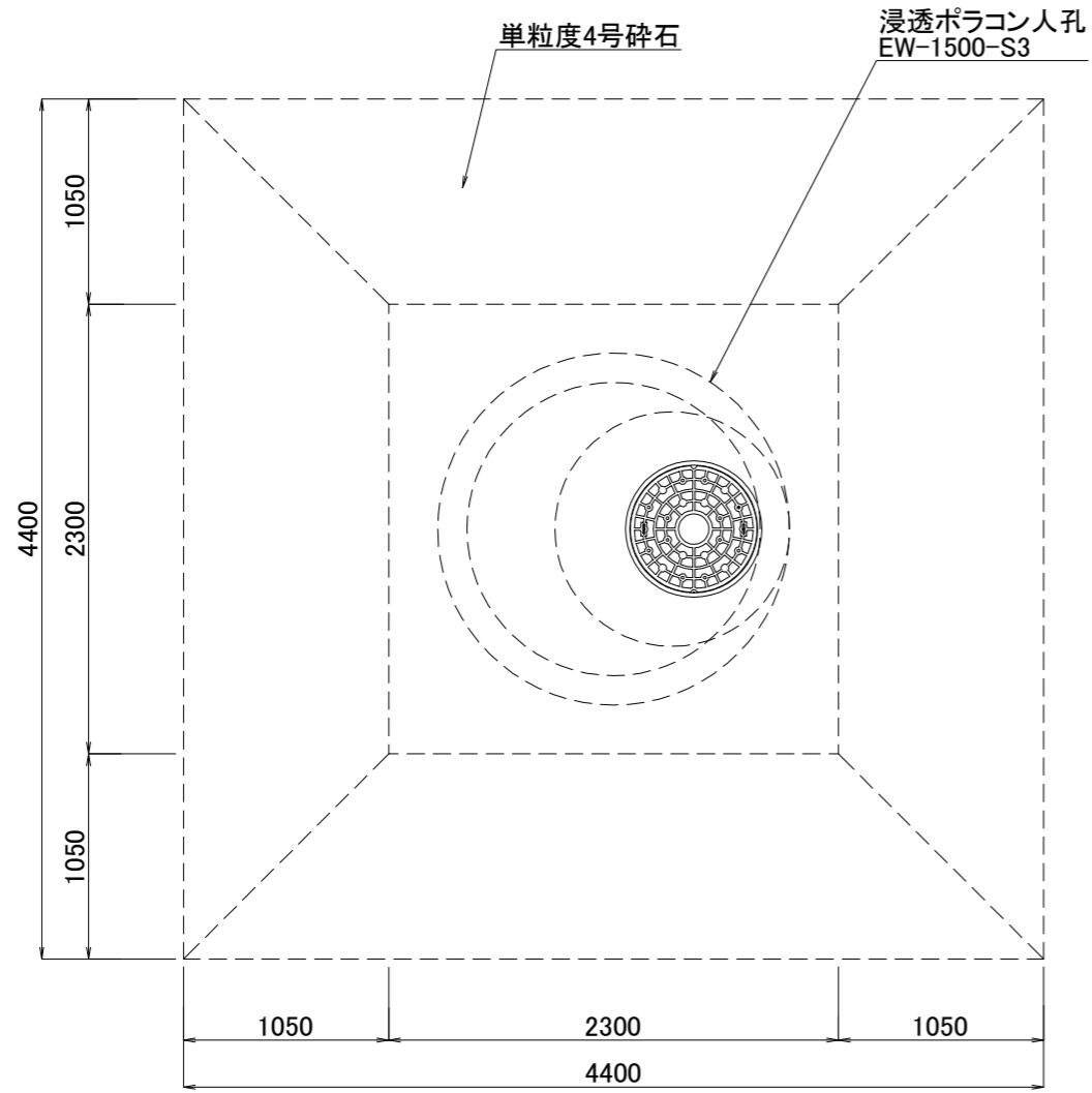
平面図
