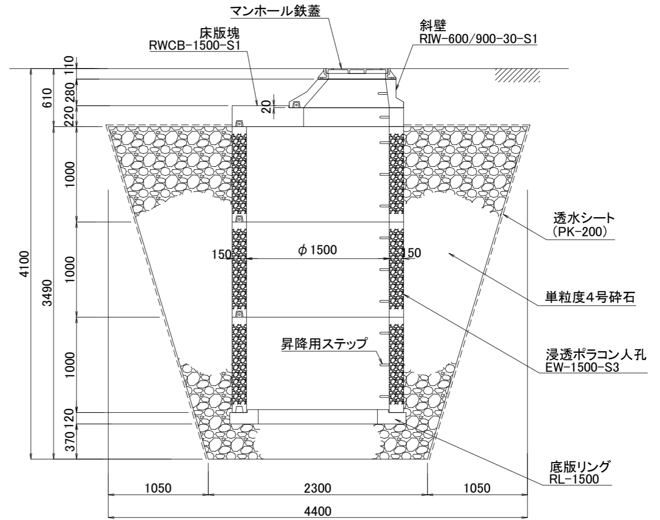
断面図
