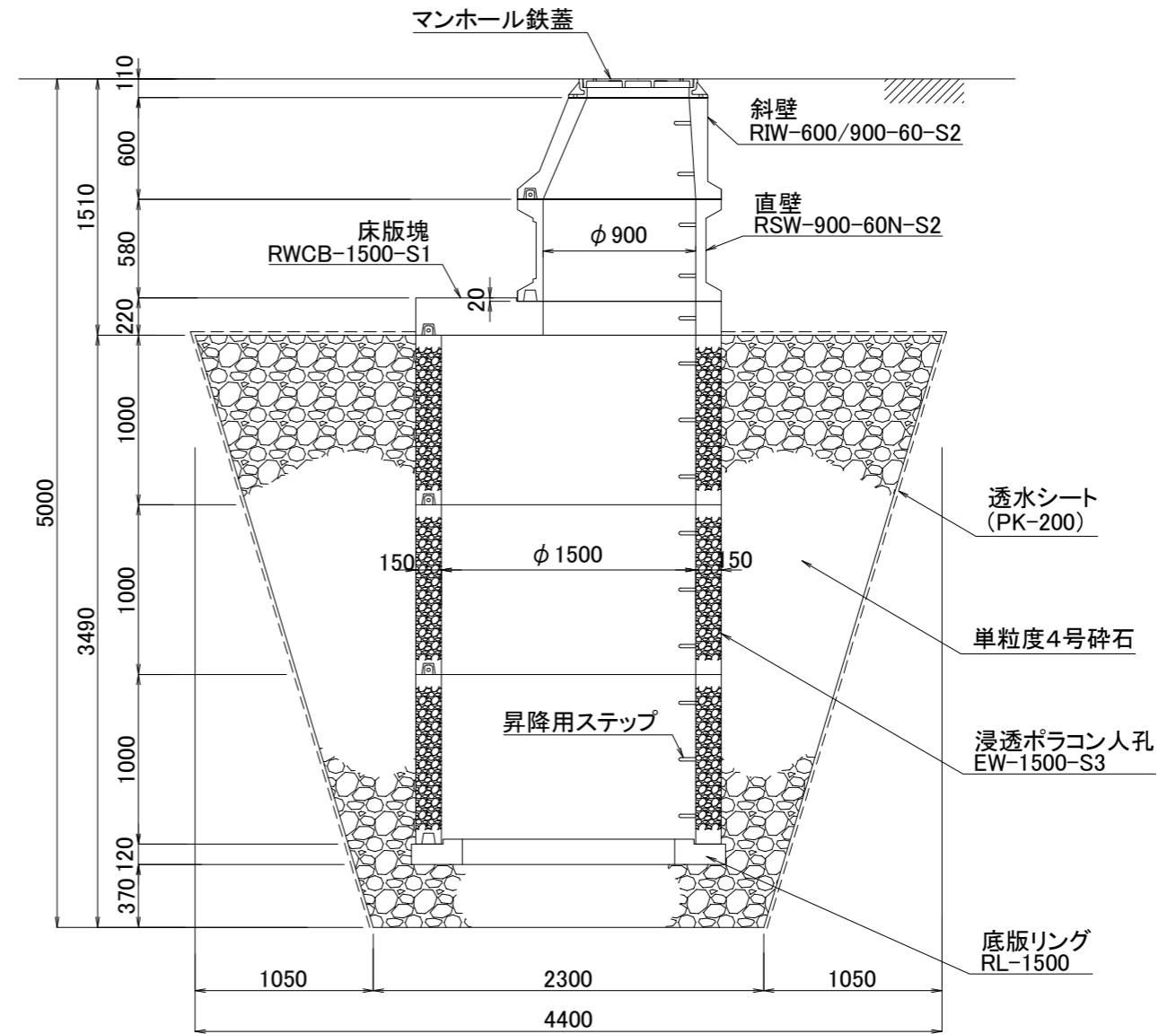
断面図
