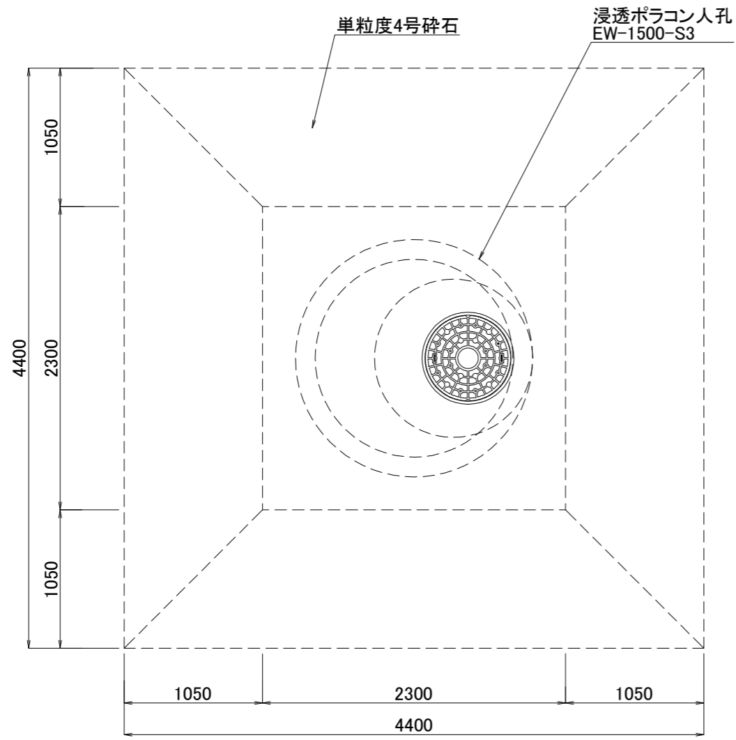
平面図
