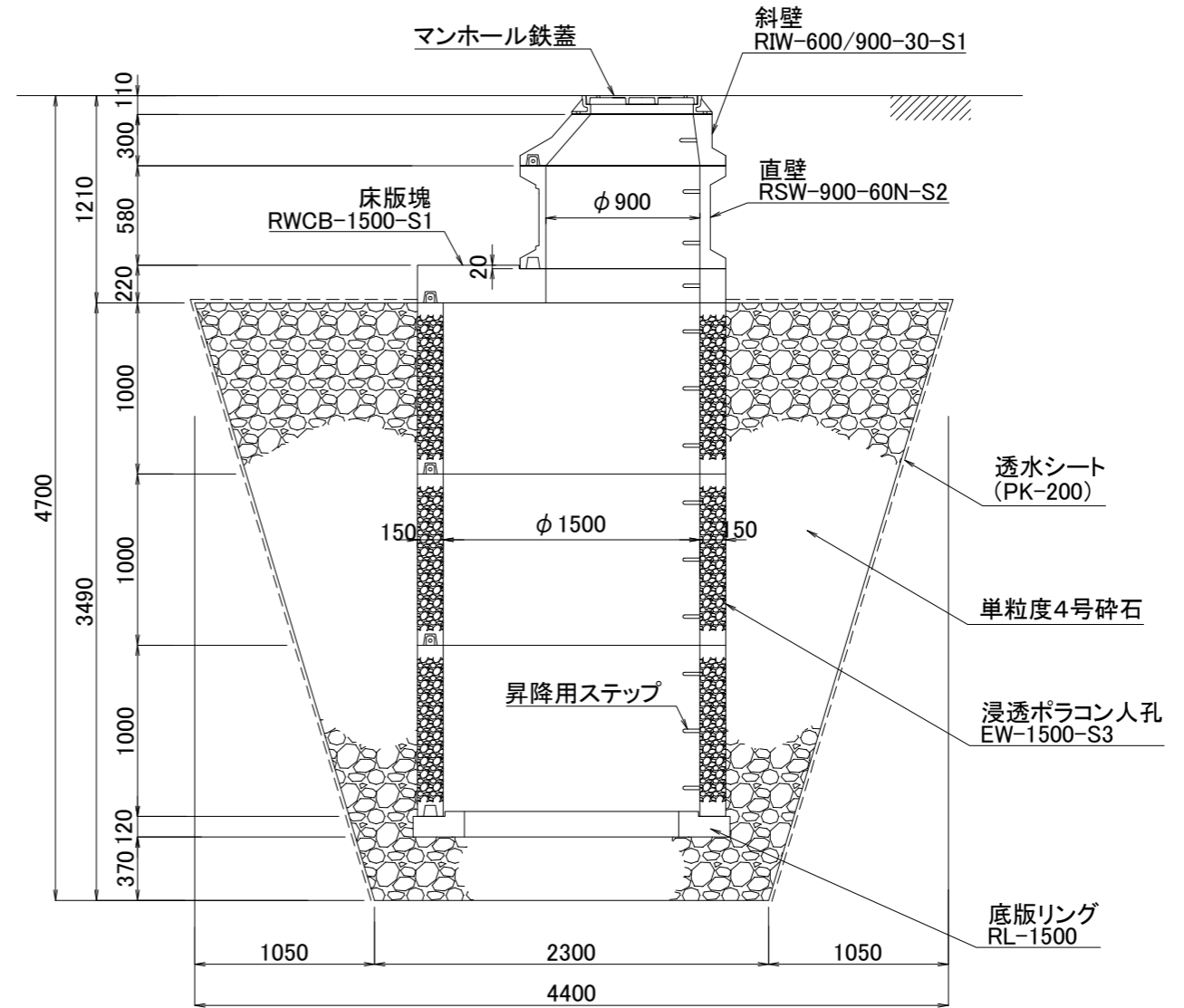
断面図
