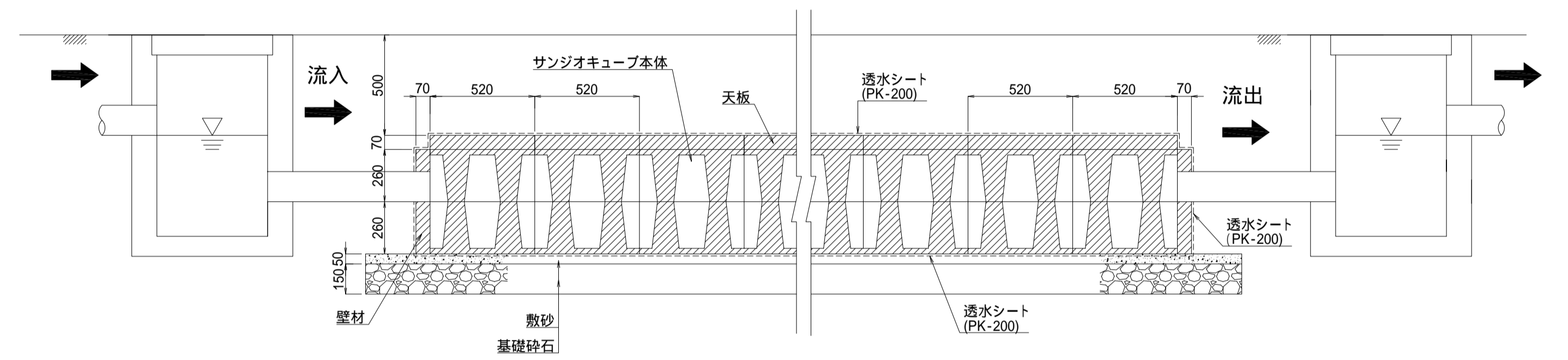
サンジोक्यूブ接続図
