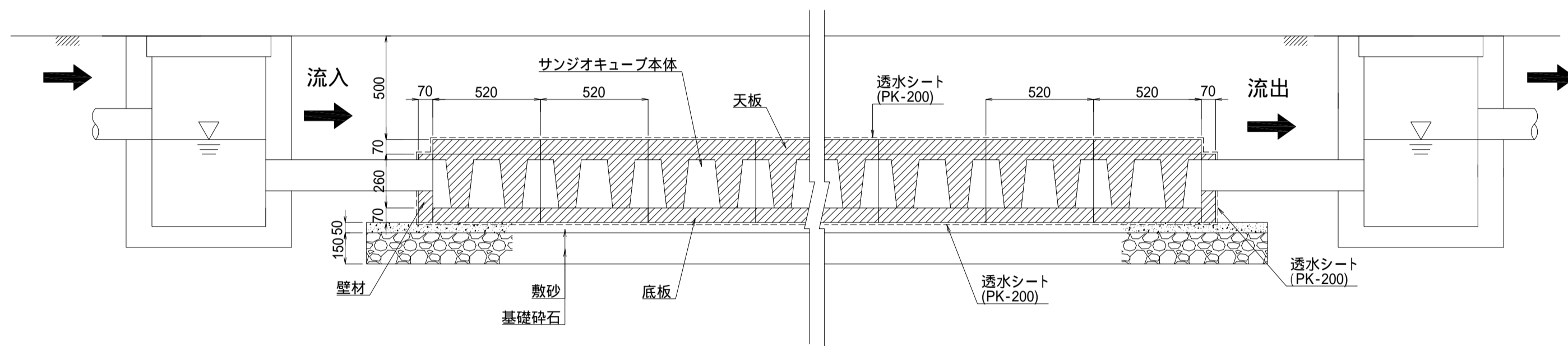
サンジोक्यूブ接続図
