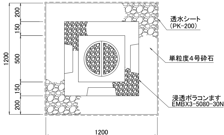
柵底部
