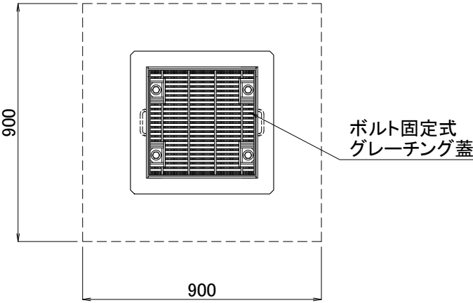
平面図
