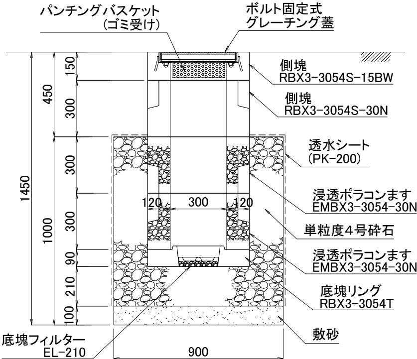
断面図
