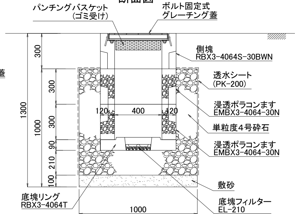
断面図
