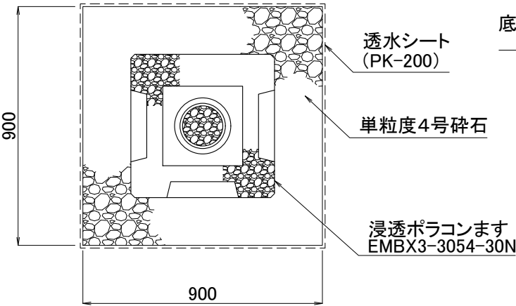
柵底部
