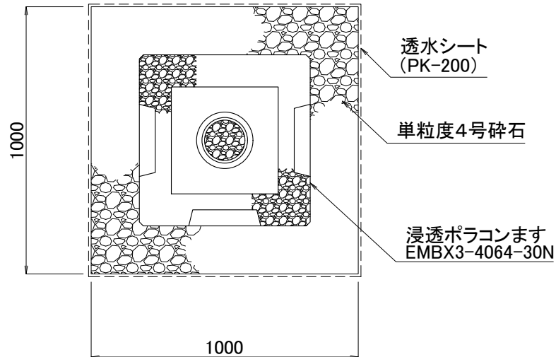
柵底部
