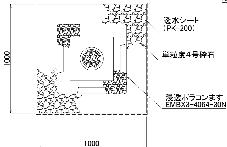
柵底部
