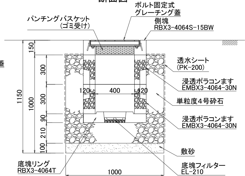
断面図
