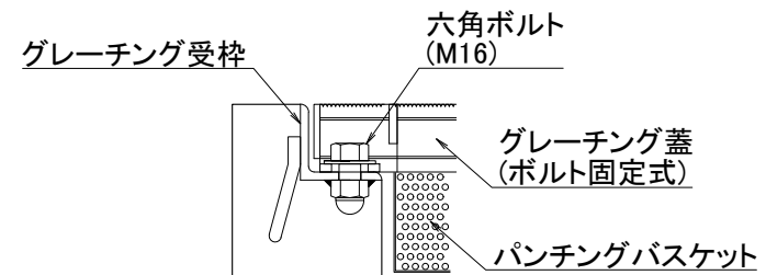
グレーチング受枠部詳細
