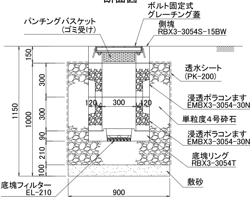
断面図
