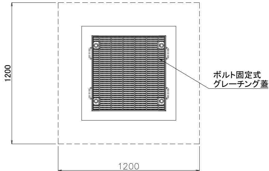
平面図
