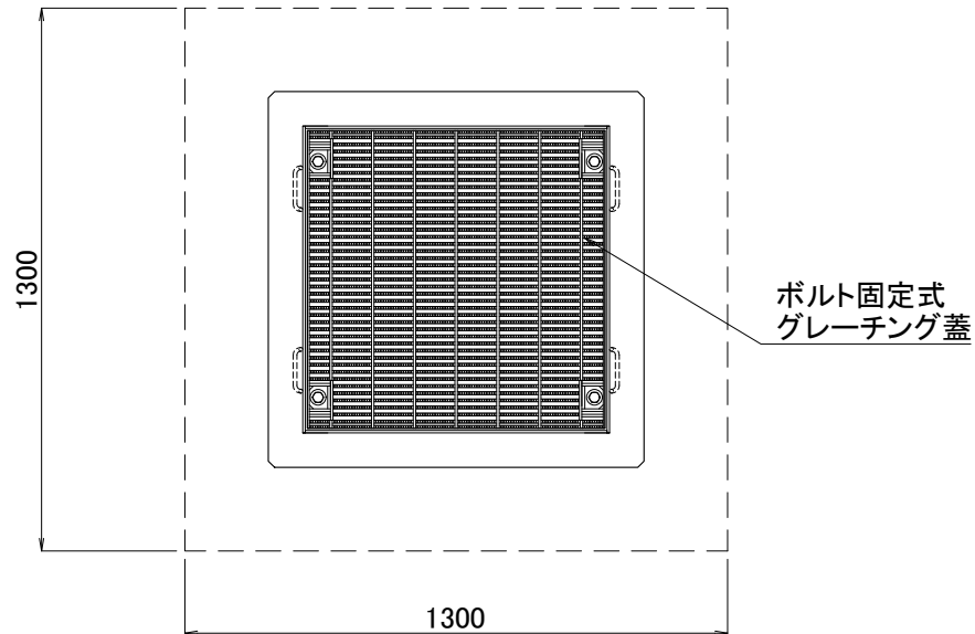
柵底部
