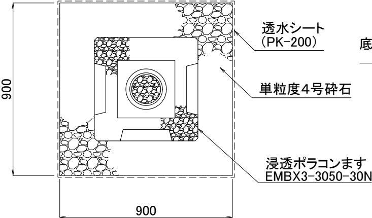
柵底部
