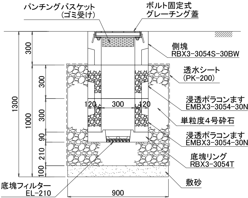
断面図
