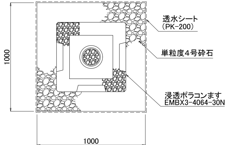
柵底部
