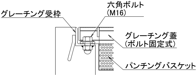
グレーチング受枠部詳細
