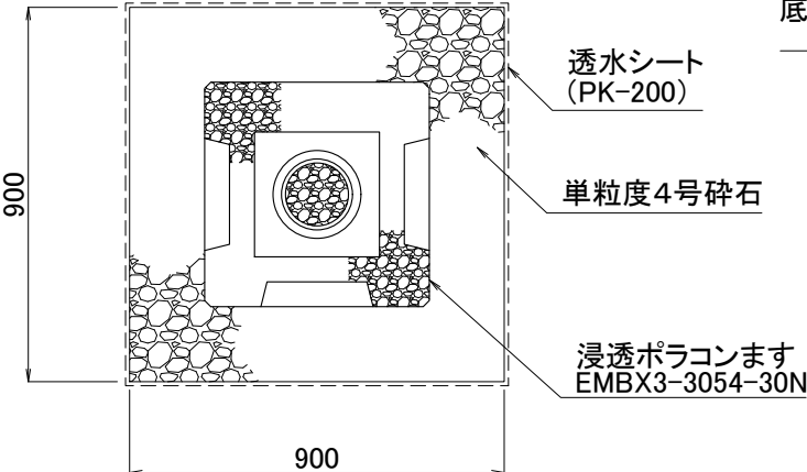
柵底部
