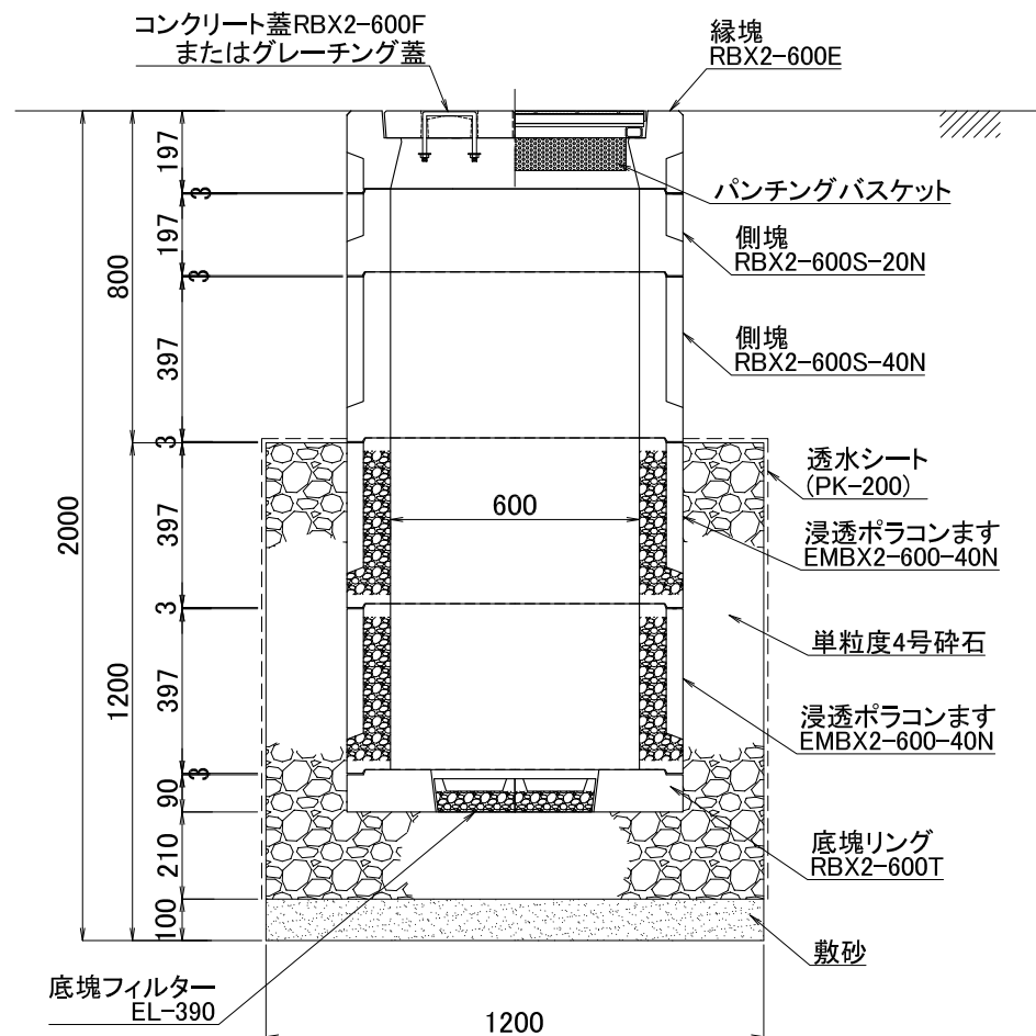
断面図
