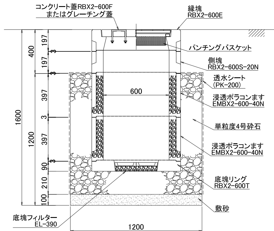
断面図
