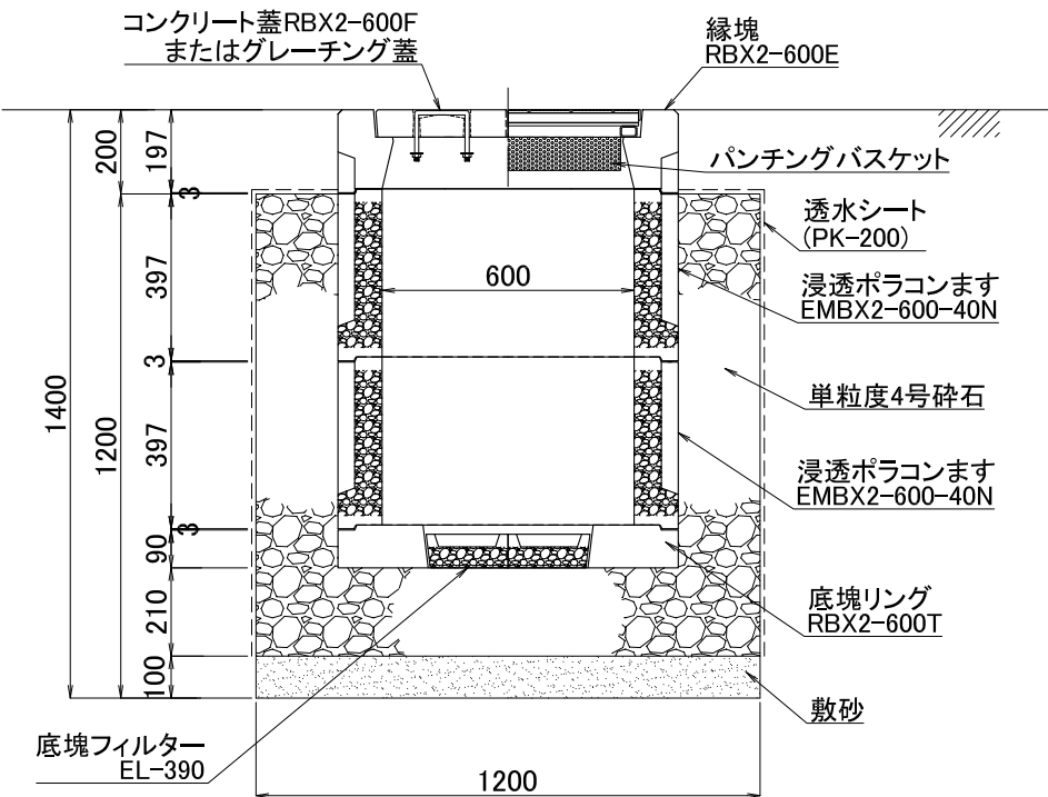
断面図
