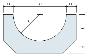
(A-A断面図)
