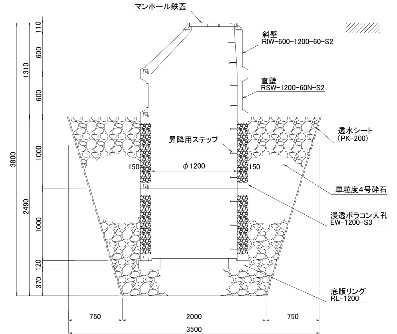
断面図
