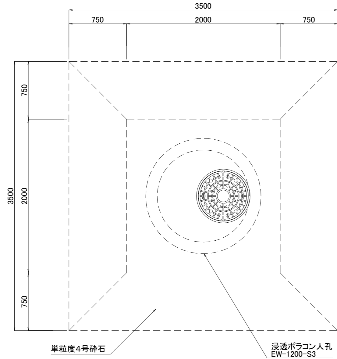
平面図
