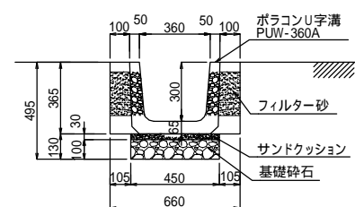
集水ポリコン側溝 PUW-360A
