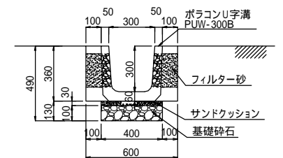
集水ポリコン側溝 PUW-300B
