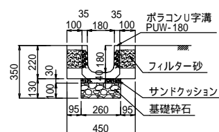
集水ポリコン側溝 PUW-180
