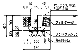
集水ポリコン側溝 PUW-240A
