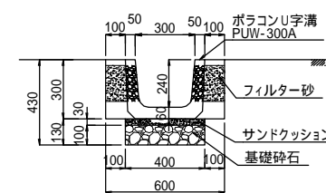
集水ポリコン側溝 PUW-300A
