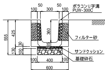
集水ポリコン側溝 PUW-300C
