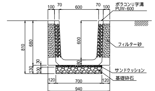
集水ポリコン側溝 PUW-600
