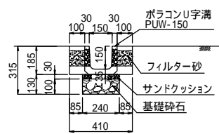
集水ポリコン側溝 PUW-150
