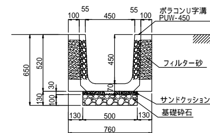
集水ポリコン側溝 PUW-450
