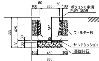
集水ポリコン側溝 PUW-360B
